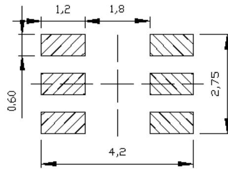
推荐焊盘
